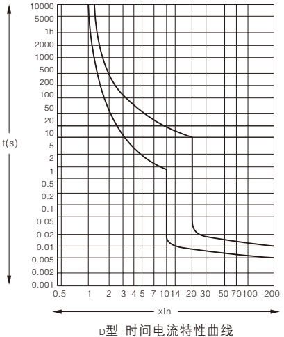
d型 时间电流特性曲线
