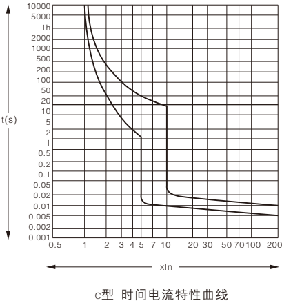
c型 时间电流特性曲线
